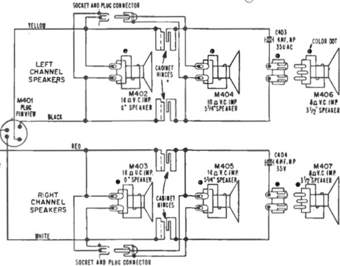
YHS 1741 SPEAKER WIRING
